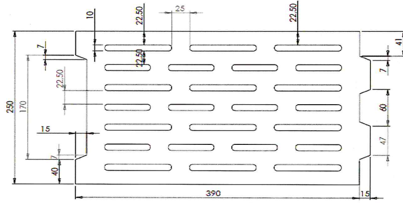
Şekil-1: TBL-25-SW Görünümü ve Ölçüleri
